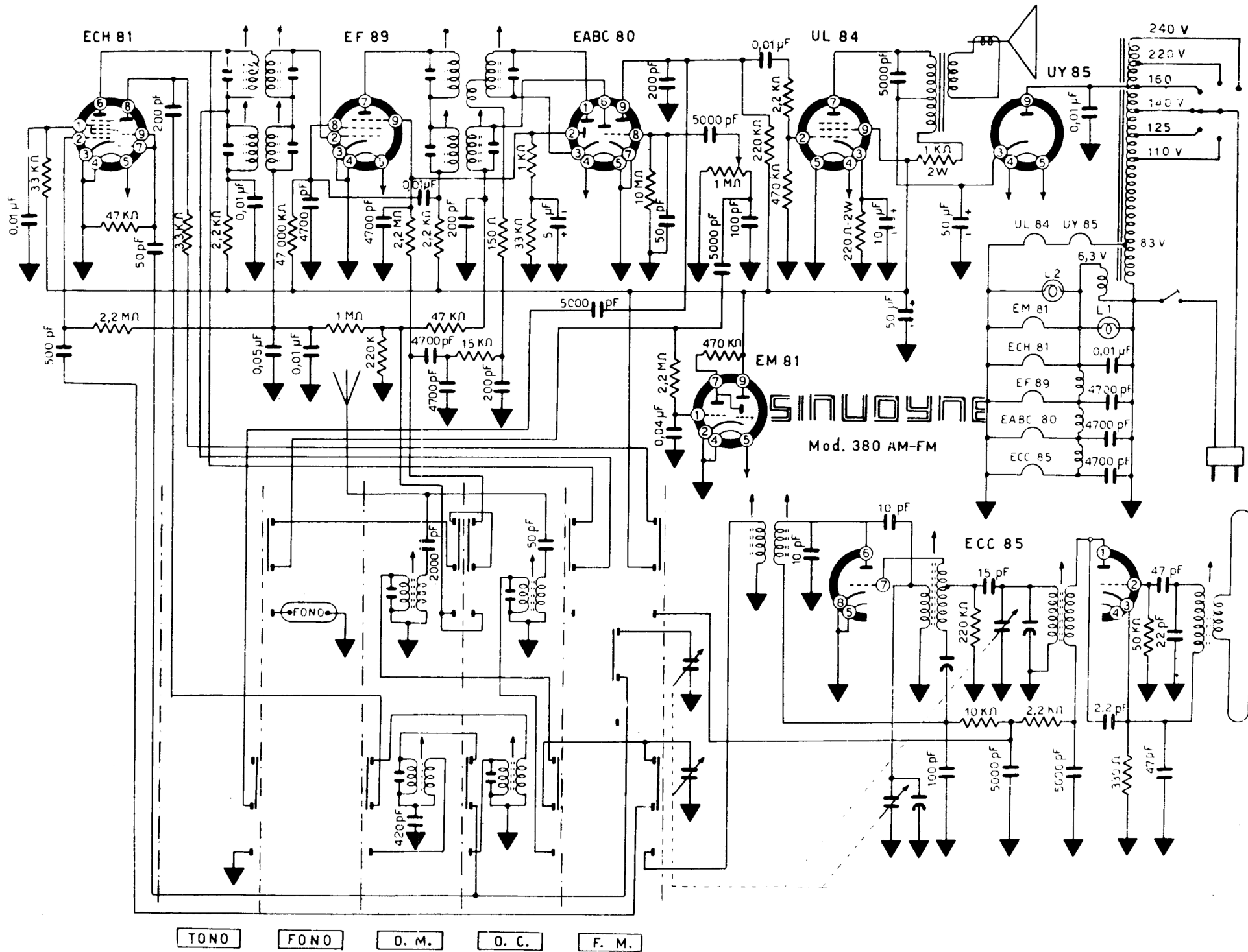
SINUDYNE - Mod. 380. Apparechio AM/FM, con una gamma onde medie, una gamma onde corte e una banda onde ultracorte, da 87 a 100,5 Mc/s. L'apparechio è provvisto di occhio magico. Media frequenza AM a 468 kc/s; media frequenza FM a 10,7 Mc/s. Resa d'uscita 2,5 watt. Consumo 50 watt.
